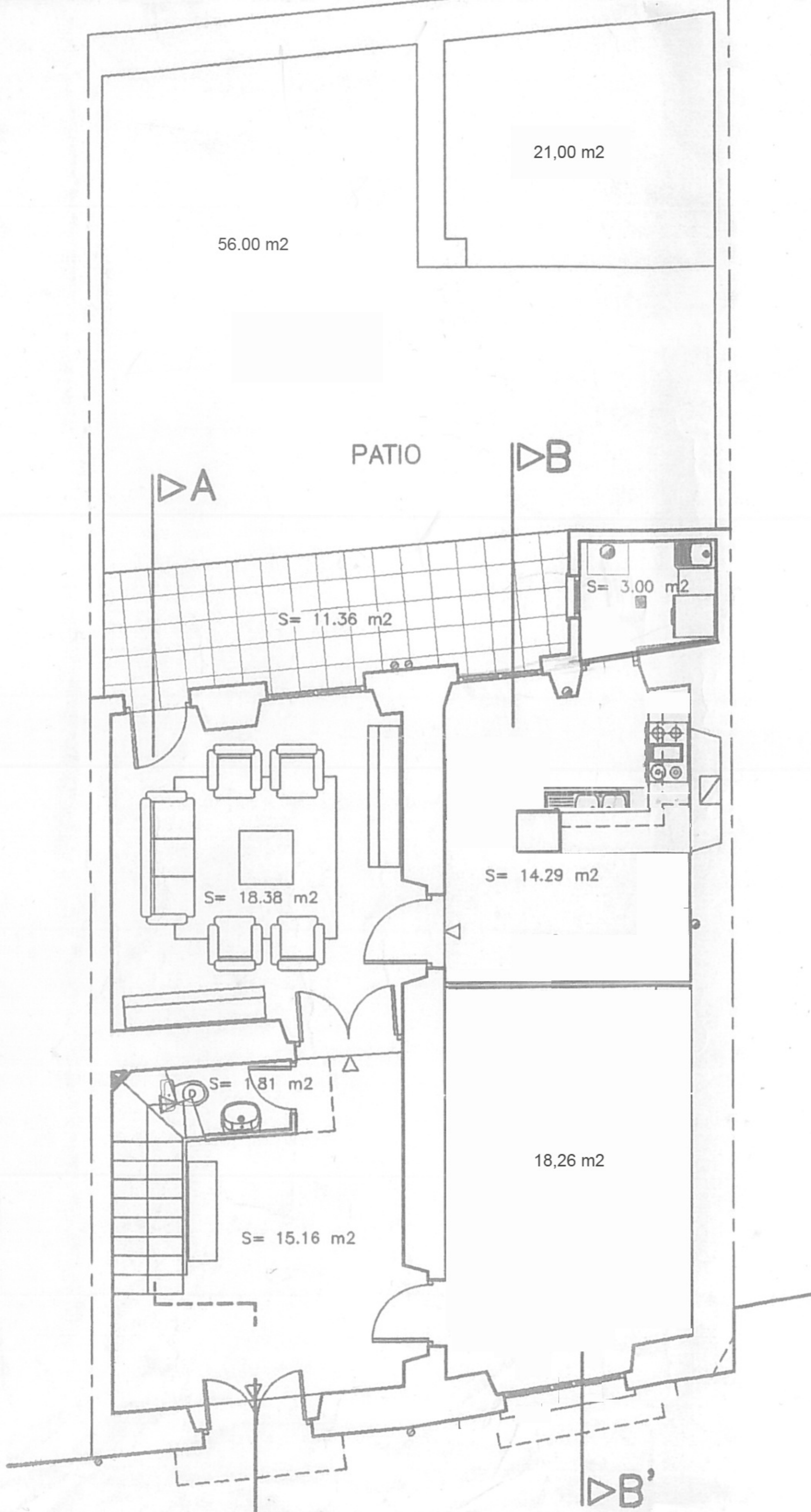
PLANTA BAJA SUP. CONSTRUIDA = 101.60 m 2 67.90
