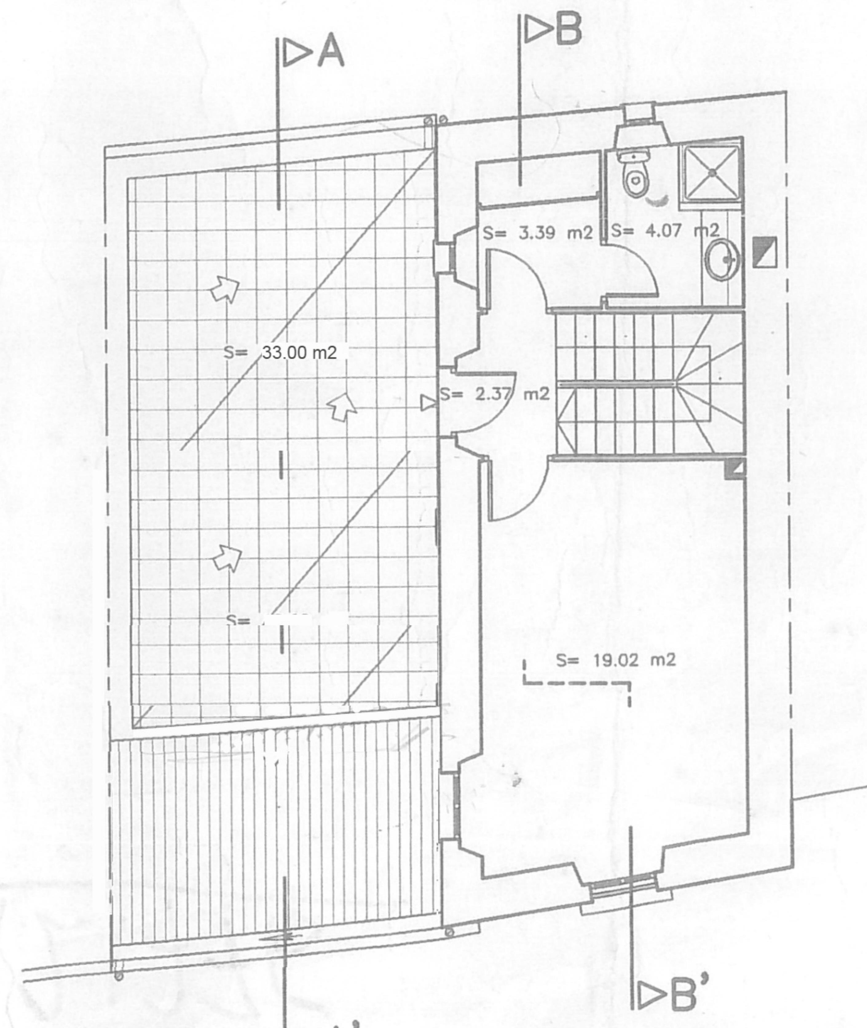
PLANTA DESVÁN SUP. CONSTRUIDA = 50.06 m 2
